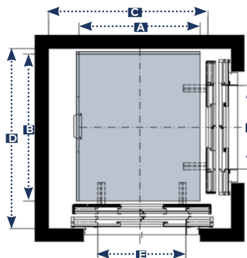
2 ACCÈS À 90° (MÉCANIQUE LATÉRALE) AVEC PORTES À 4VC
