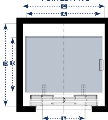
SIMPLE ACCÈS (MÉCANIQUE EN FOND DE GAINÉ) AVEC PORTES À 4VC
