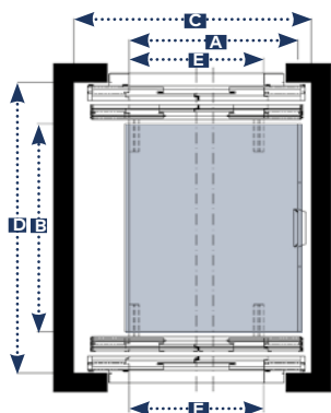
2 ACCÈS À 180° (MÉCANIQUE LATÉRALE) AVEC PORTES À 4VC
