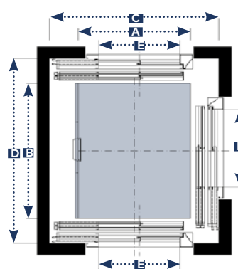
TRIPLE ACCÈS (MÉCANIQUE LATÉRALE) AVEC PORTES À 2VT
