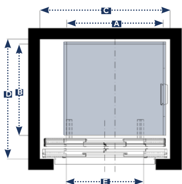
SIMPLE ACCÈS (MÉCANIQUE LATÉRALE) AVEC PORTES À 4VC
