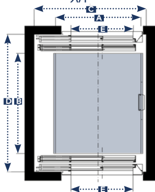
2 ACCÈS À 180° (MÉCANIQUE LATÉRALE) AVEC PORTES À 2VT
