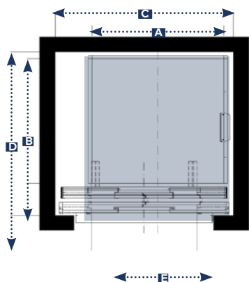
SIMPLE ACCÈS (MÉCANIQUE LATÉRALE) AVEC PORTES À 2VT
