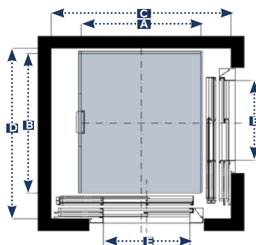
2 ACCÈS À 90° (MÉCANIQUE LATÉRALE) AVEC PORTES À 2VT
